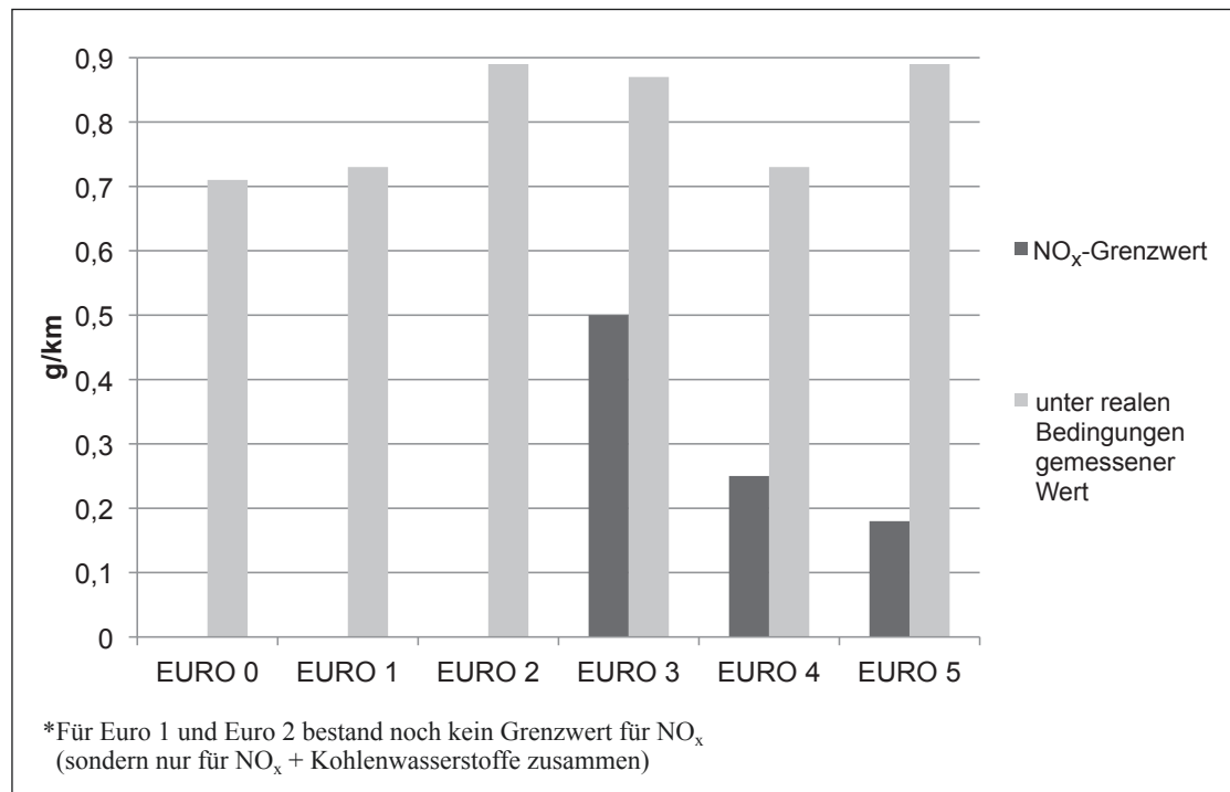
Zulässige (Grenzwert*) und unter realen Fahrbedingungen gemessene Stickstoffoxidemissionen bei Diesel-Pkw verteilt über bestehende Euro-Standards
