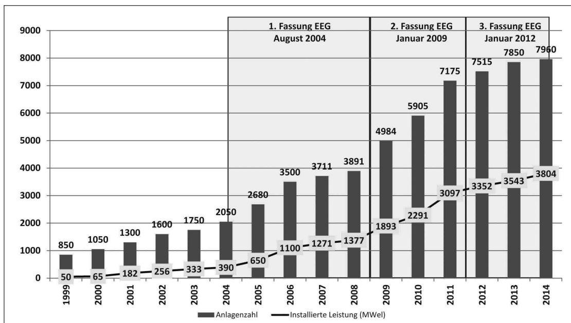
Anzahl der Biogasanlagen und installierte Leistung
