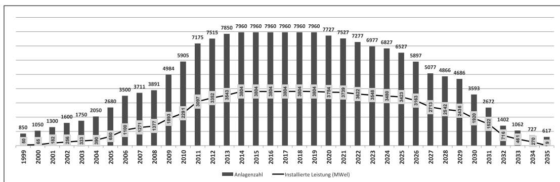
Entwicklung der nach EEG vergüteten Biogasanlagen und installierter Leistung (Inbetriebnahme 1999 bis 2014)
