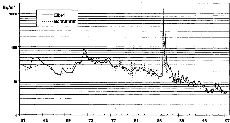
Fig. 1: Zeitlicher Verlauf der Cs-137 Konzentration ( \text{Bq/m}^3 ) an den Positionen der ehemaligen Feuerschiffe Borkumriff und Elbe 1.
